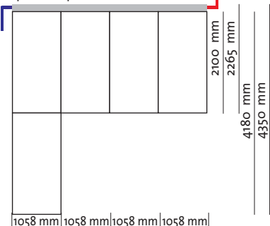
Kombination topSol und topSol doho
